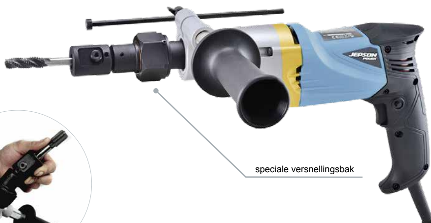
Flexibele draadhouder
